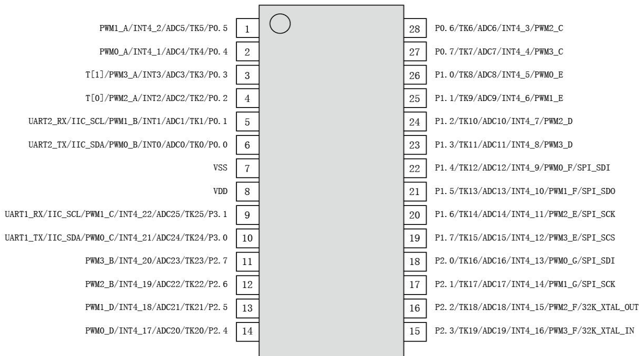
图 5-1-1 SOP28 封装引脚图
