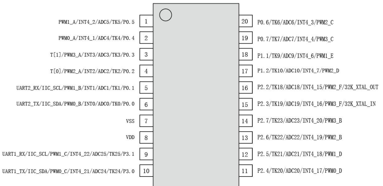
图 5-1-4 SOP20 封装引脚图
