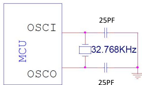
图 9-1-4-1 XOSCL 典型电路图
