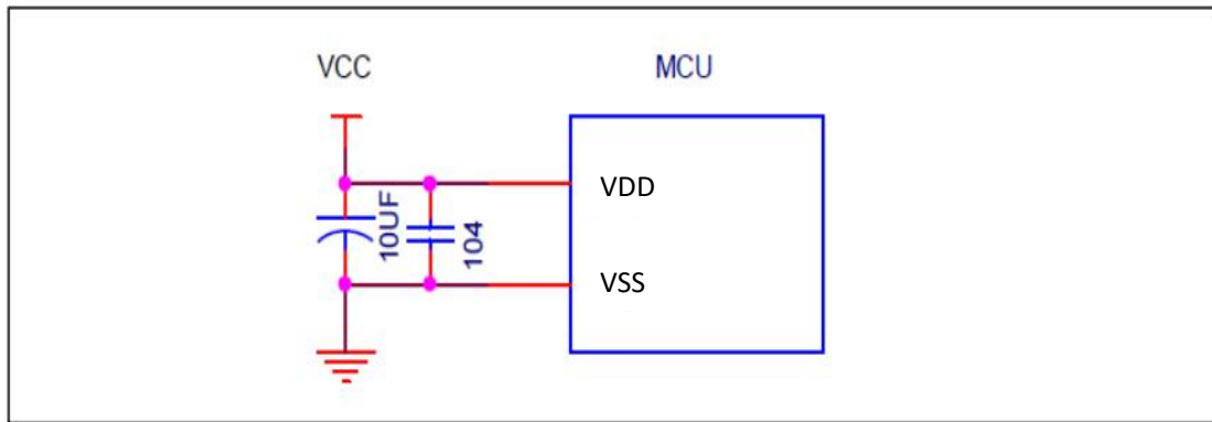
图 10-1-1 芯片供电典型电路图
