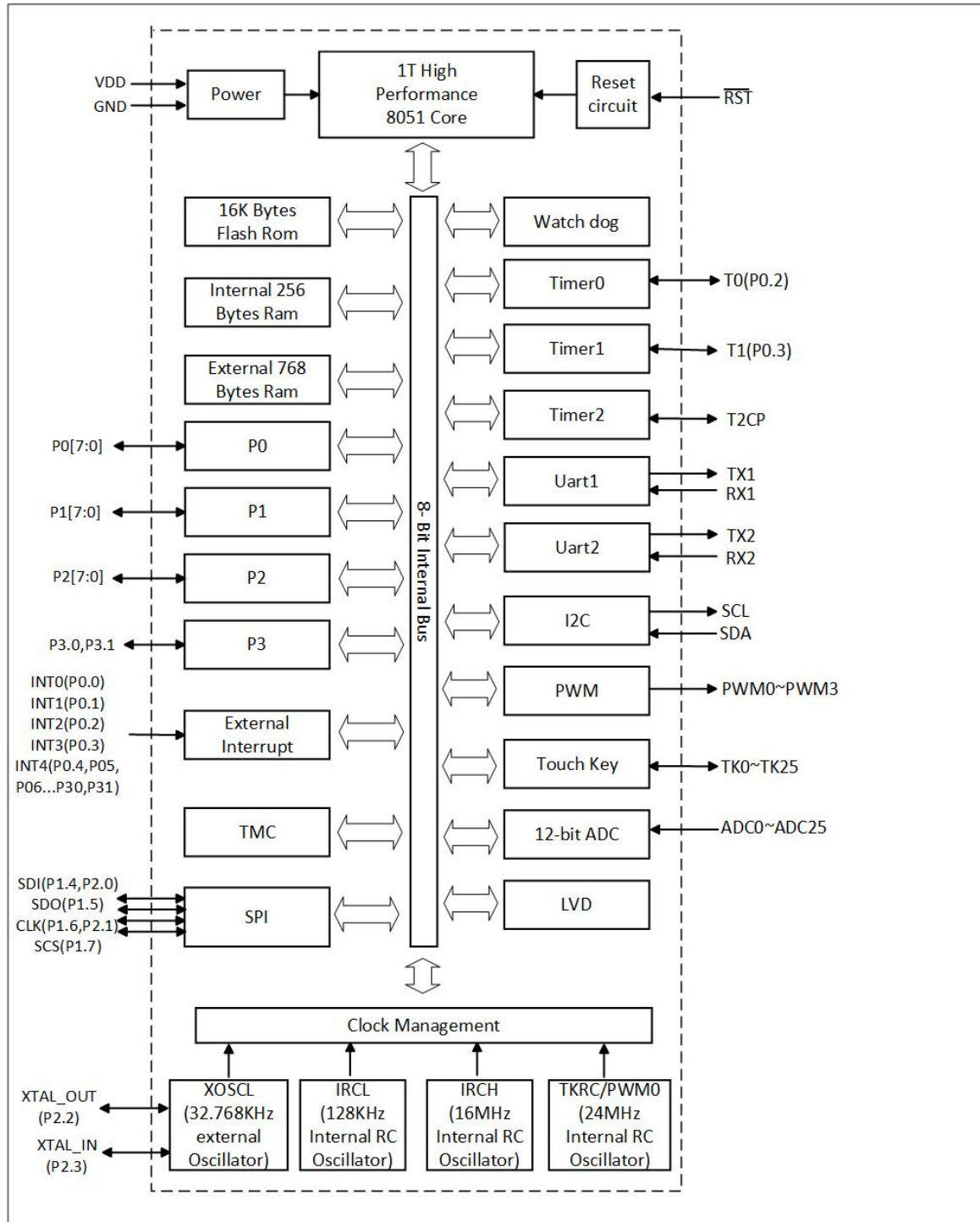
图 4-1-1 芯片框图
