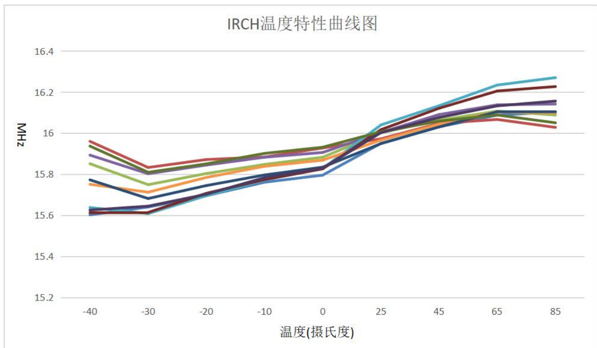
图 23-5-1 IRCH 温度特性曲线图
