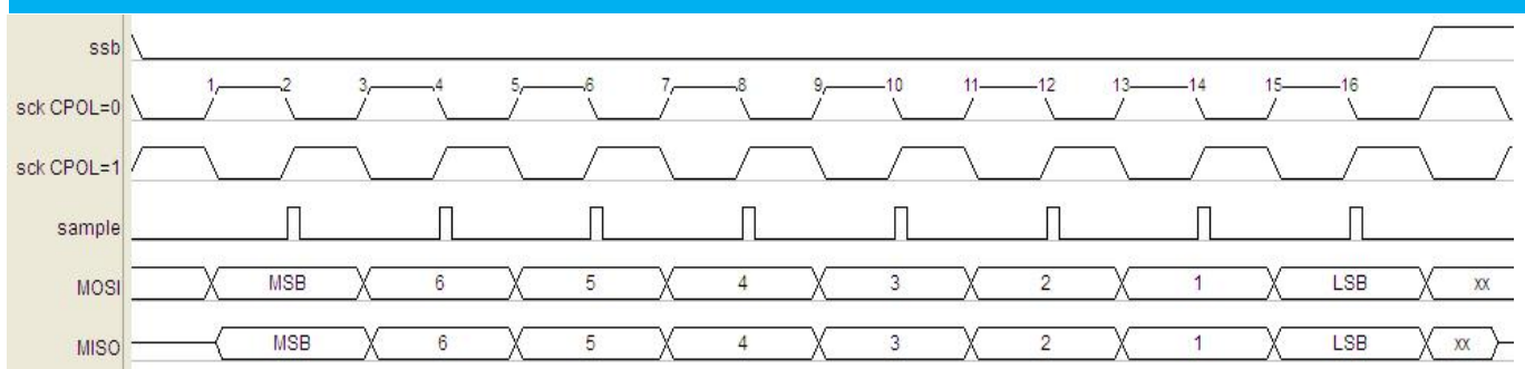
图 19-1-4 CPHA=1 时 SPI 时序图
